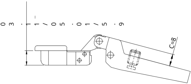
CODO 9
