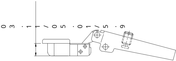
CODO 0
